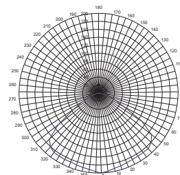
ЖСП-07У-70
